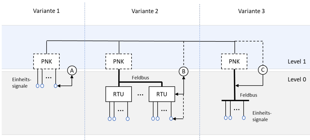
Abbildung 6 Ansteuerung von Feldsignalen
