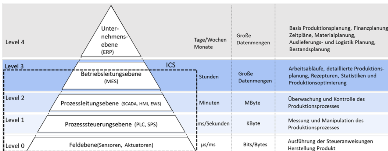
Abbildung 3 Hierarchische Ebenen der Produktionspyramide (8)
